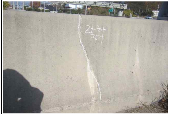
연석 균열(cw:0.3mm이상) (25년 하반기 정기안전점검)
