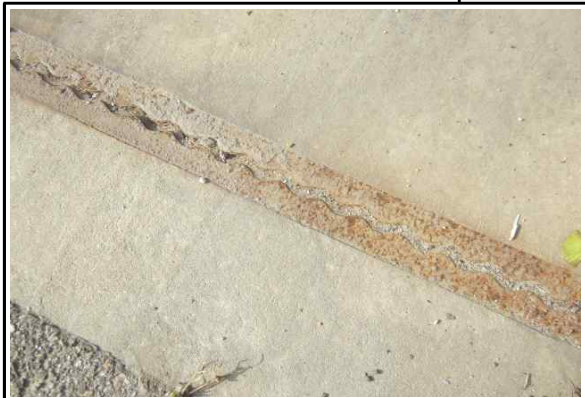
신축이음 유간 토사퇴적 (25년 하반기 정기안전점검)
