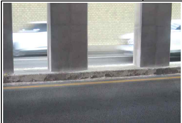
Sta. 100(강화) 연석-탄산화방지재 박리 (25년 하반기 정기안전점검)
