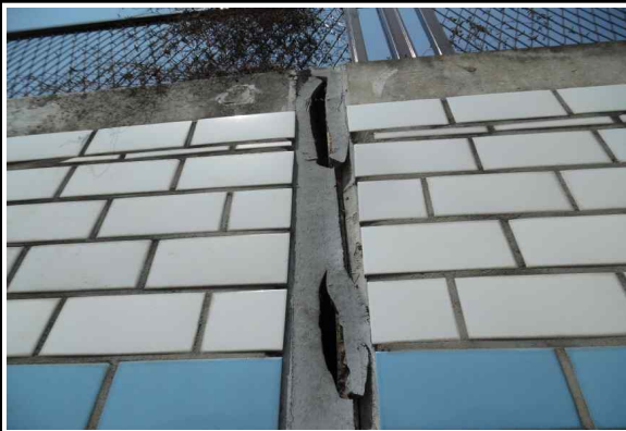
U-Type구간 실런트 파손 (25년 상반기 정기안전점검)
