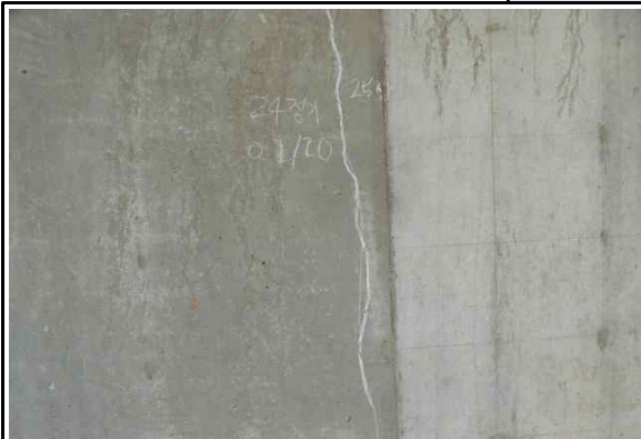
교대 균열(cw:0.3mm미만) (25년 상반기 정기안전점검)
