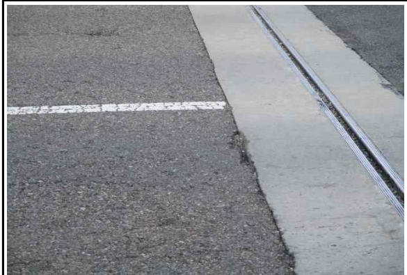
교면포장 접속부 아스콘 파손 (25년 하반기 정기안전점검)
