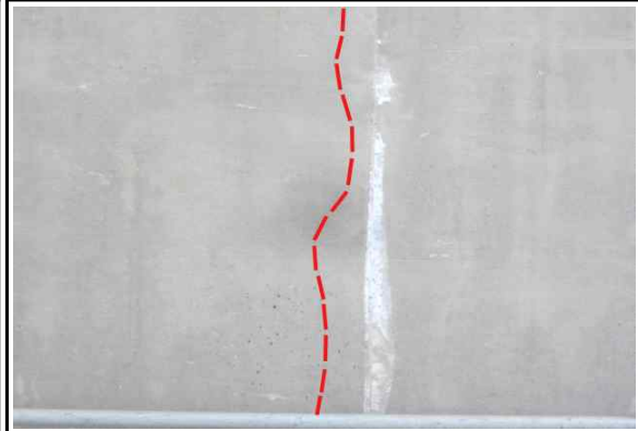
바닥판하면 균열(cw:0.3mm미만) (25년 하반기 정기안전점검)
