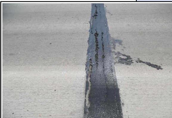
포장부 조인트 파손 (25년 상반기 정기안전점검)
