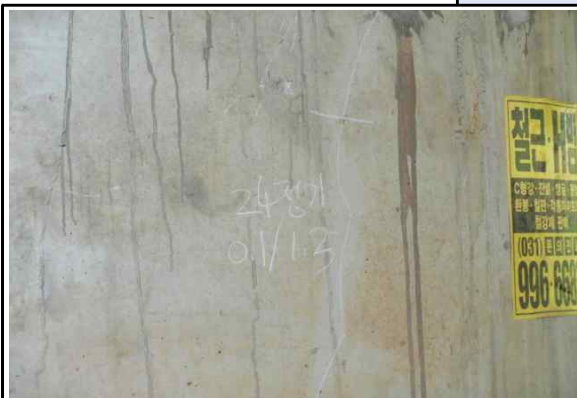
교각 균열(cw:0.3mm미만) (25년 상반기 정기안전점검)
