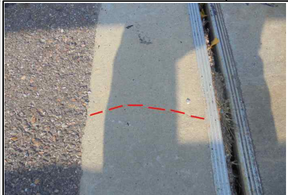
P2 신축이음-후타재 균열(cw:0.3mm미만) (25년 하반기 정기안전점검)
