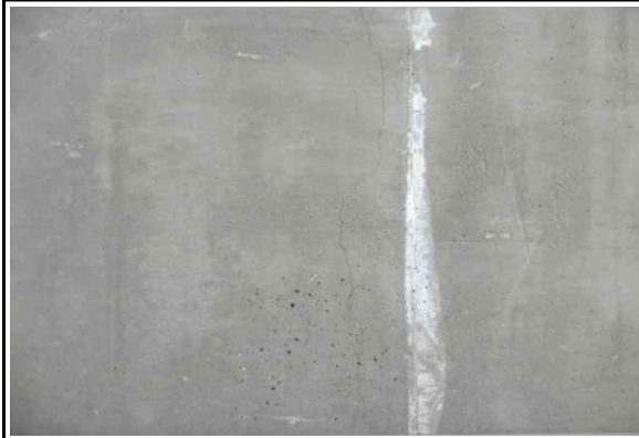
바닥판하면 균열(cw:0.3mm미만) (25년 상반기 정기안전점검)
