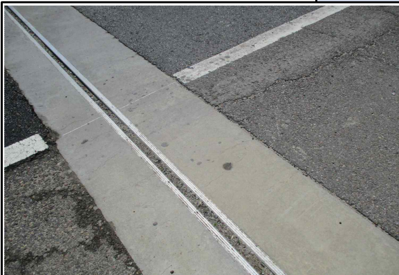
A1 신축이음-후타재 균열(cw:0.3mm미만) (25년 상반기 정기안전점검)
