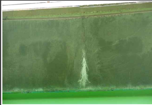
S1 캔틸레버-균열부 백태 (25년 상반기 정기안전점검)
