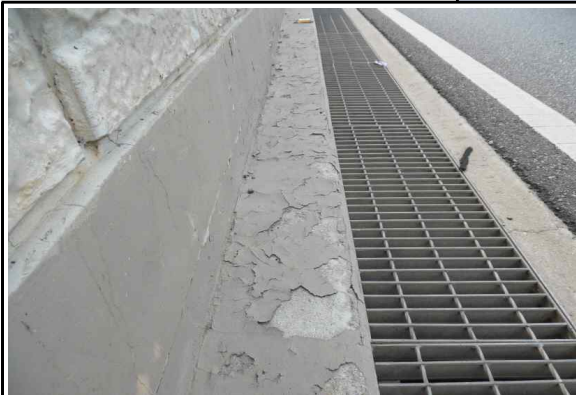
Sta. 002(서울) 연석-탄산화방지재 박리 (25년 상반기 정기안전점검)
