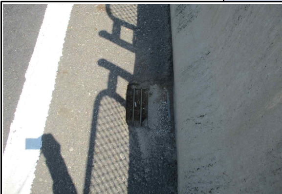
S2 배수시설-배수구 막힘 (25년 상반기 정기안전점검)
