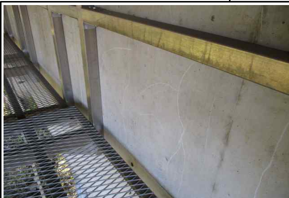
교각 망상균열(cw:0.3mm미만) (25년 하반기 정기안전점검)
