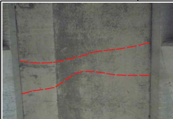
바닥판하면 균열(cw:0.3mm미만) (25년 하반기 정기안전점검)
