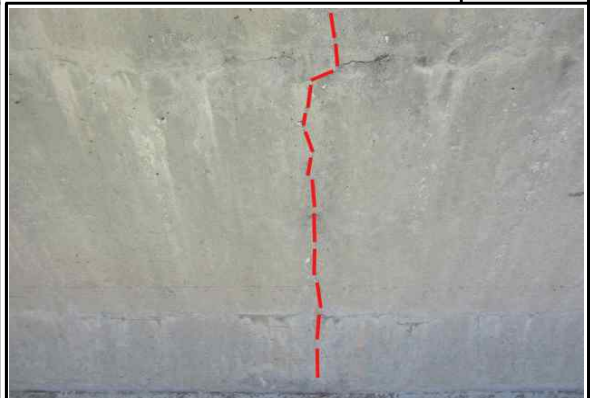
S2 방호울타리-균열(cw:0.3mm미만) (25년 하반기 정기안전점검)
