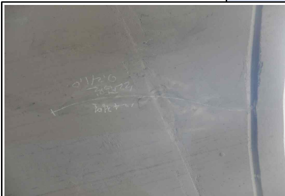
BOX 상부슬래브 하면-균열(cw:0.3mm미만) (25년 상반기 정기안전점검)
