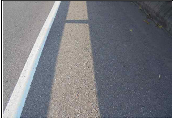
S4 교면포장-포장균열 (25년 하반기 정기안전점검)
