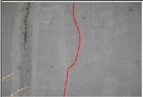
교대 균열(cw:0.3mm미만) (25년 하반기 정기안전점검)
