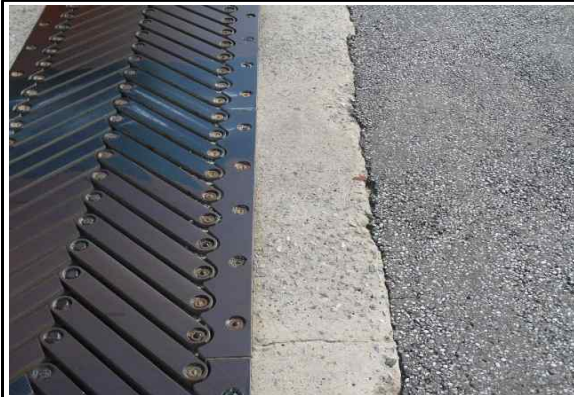
P8(강화) 신축이음-후타재 균열 (25년 상반기 정기안전점검)
