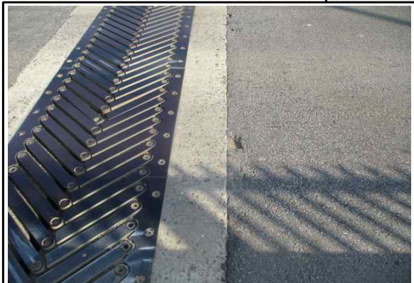
S9(서울) 교면포장-파손 (25년 하반기 정기안전점검)
