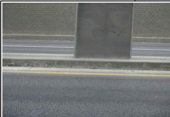
Sta. 100(강화) 연석-탄산화방지재 박리 (25년 상반기 정기안전점검)
