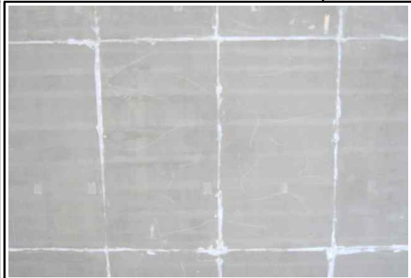
바닥판하면 망상균열(cw:0.3mm미만) (25년 하반기 정기안전점검)
