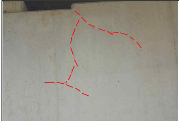
P3 코핑(배면)-망상균열(cw:0.3mm미만) (25년 하반기 정기안전점검)
