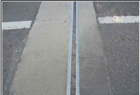
A1 신축이음-유간 토사퇴적 (25년 하반기 정기안전점검)
