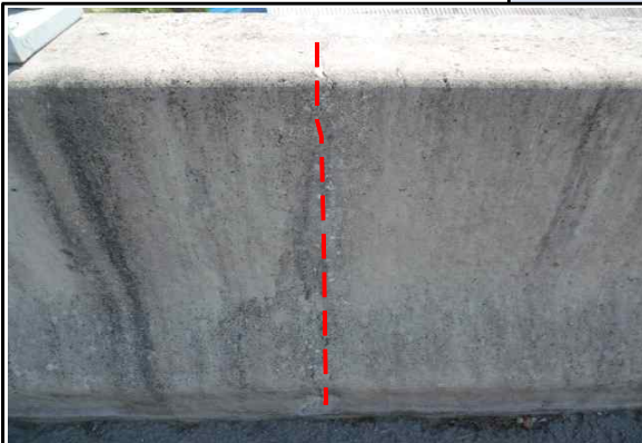
S2 방호벽-균열(cw:0.3mm미만) (25년 상반기 정기안전점검)
