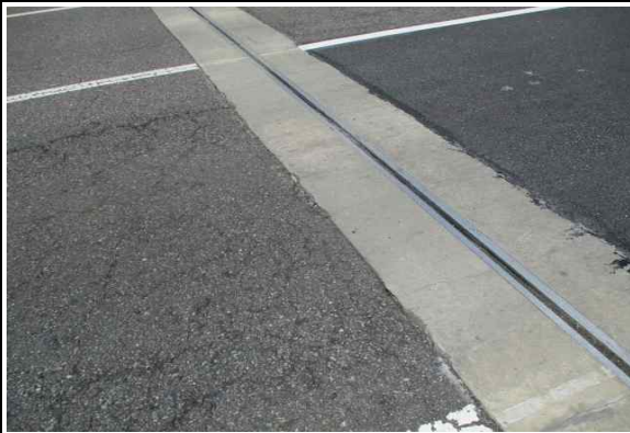
신축이음 후타재 파손 (25년 상반기 정기안전점검)
