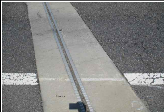
신축이음 후타재 균열(cw:0.3mm미만) (25년 상반기 정기안전점검)
