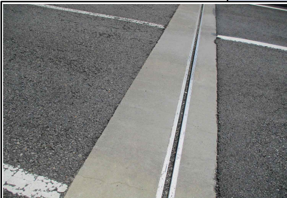
A2 신축이음-후타재 균열(cw:0.3mm미만) (25년 상반기 정기안전점검)
