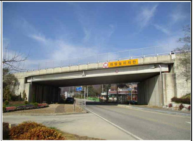
측면 전경
