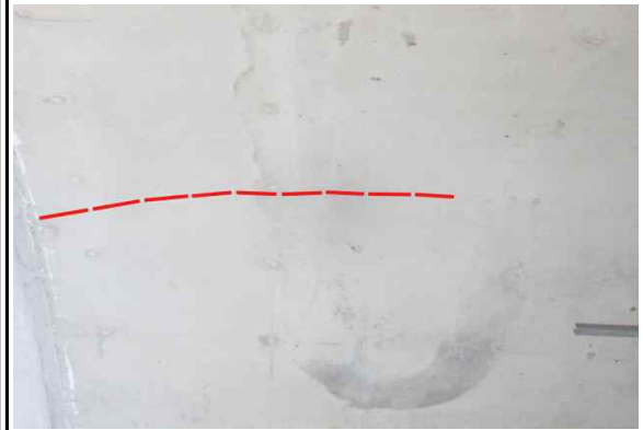
시점(Span 2) 갭문-균열(cw:0.3mm미만) (25년 하반기 정기안전점검)
