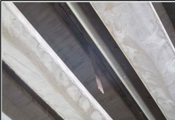
S2 바닥판하면-완충재 탈락 (25년 상반기 정기안전점검)
