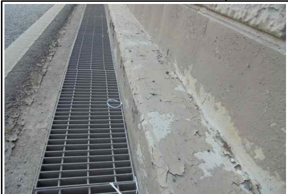
Sta. 002(서울) 연석-탄산화방지재 박리 (25년 하반기 정기안전점검)
