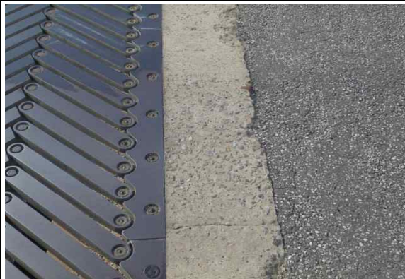
P8(강화) 신축이음-후타재 마모 (25년 하반기 정기안전점검)
