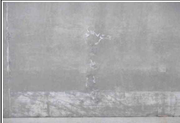
바닥판하면 균열부 백태(cw:0.3mm미만) (25년 상반기 정기안전점검)
