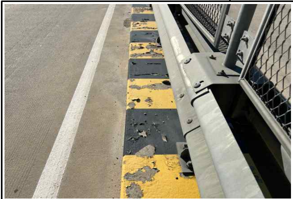
중앙분리대 연석 도장박리 (25년 하반기 정기안전점검)
